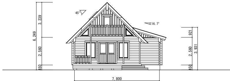
立面图 S=1/100
