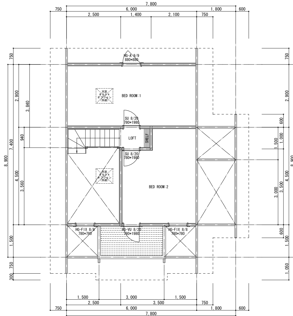
2階平面図 S=1/50
