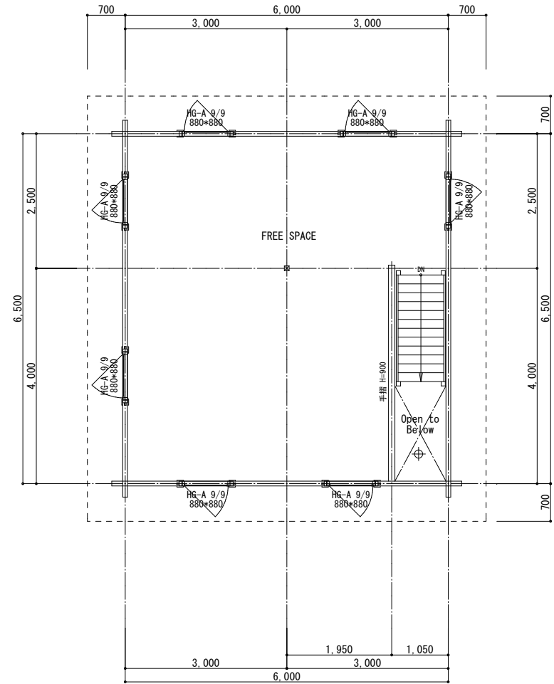
2 階平面図 S=1/50
