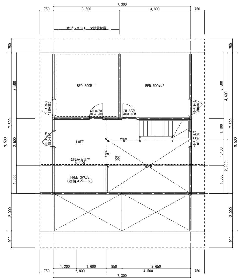
2階平面図 S=1/50
