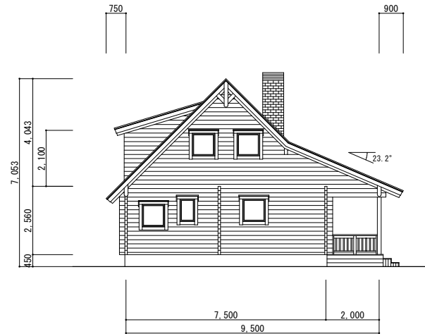
立面图 S=1/100
