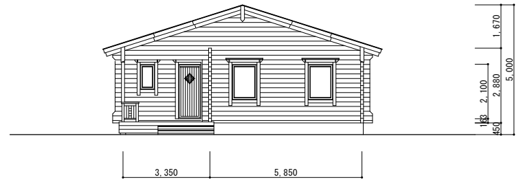
立面图 S=1/100
