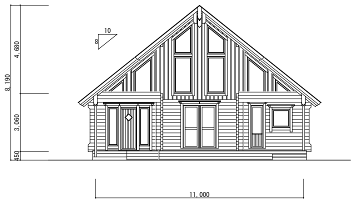
立面图 S=1/100
