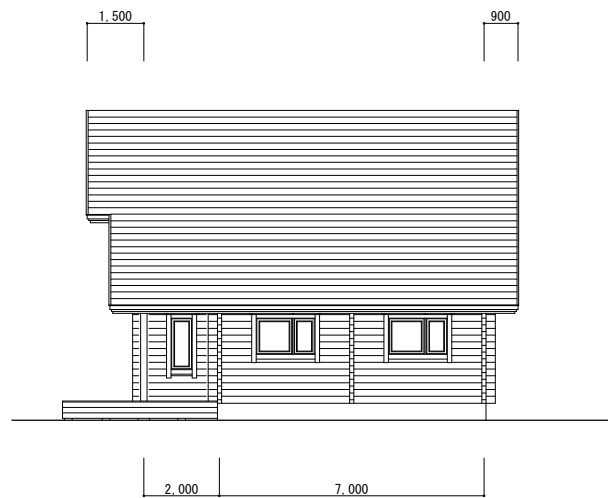
立面图 S=1/100
